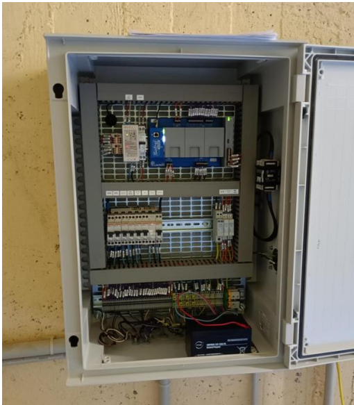
Exemple : Renouvellement armoire télégestion réservoir de Brémencourt
